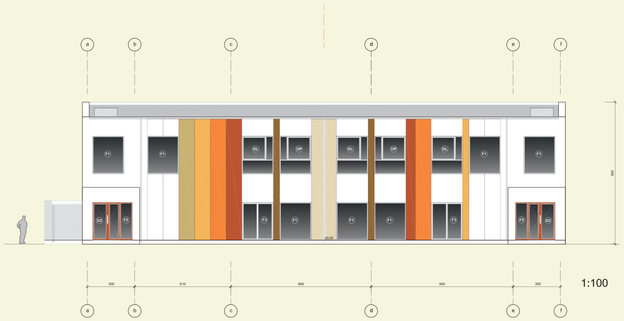
ELEWACJA POŁUDNIOWA
